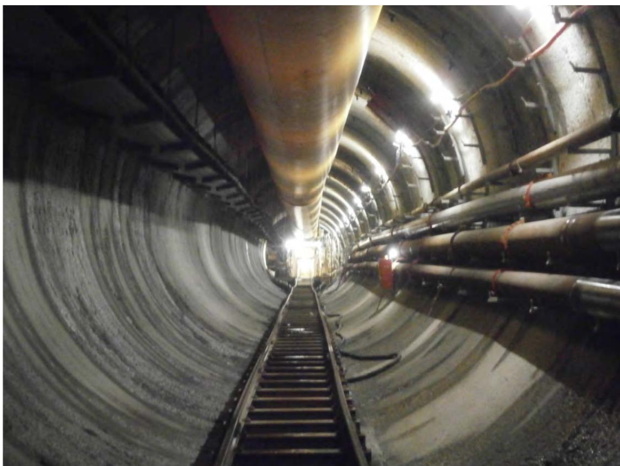
LTF - chantier de La Maddalena : Vue de la galerie dans les micaschistes du complexe de Clarea
